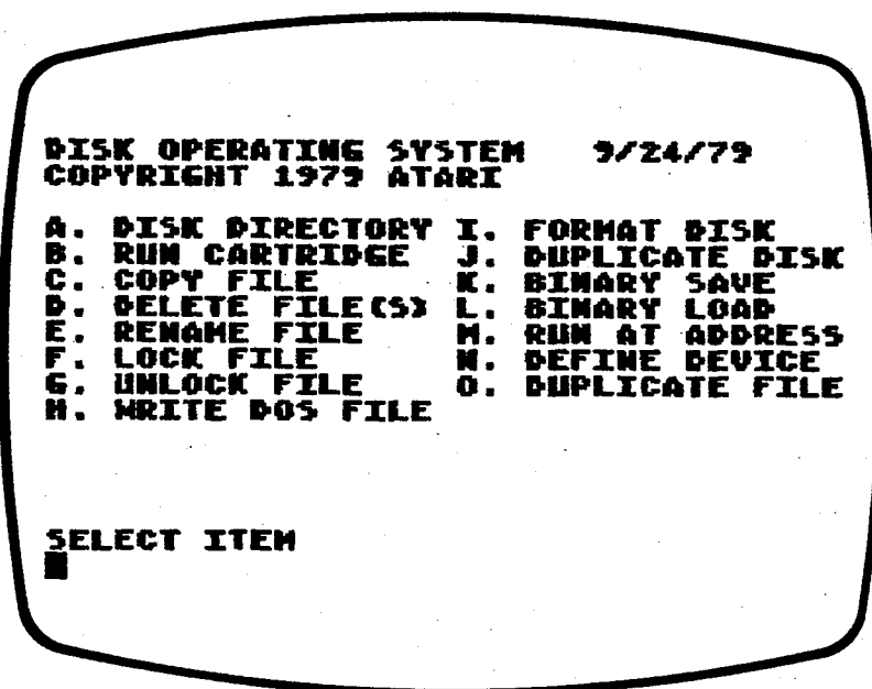
FIGURE 5-1. DOS MENU
